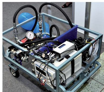
Elektro-mechanické zariadenie tímu vývojárov z Technickej fakulty, určené na testovanie hydraulického okruhu pracovnej hydrauliky
